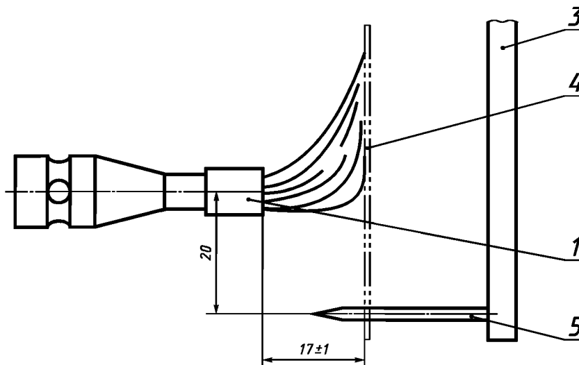
в — рабочее положение горелки при испытании
